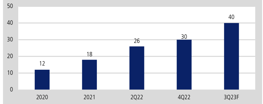
圖 1: ABF 月產能將於 2023 年擴增至 4000 萬顆
